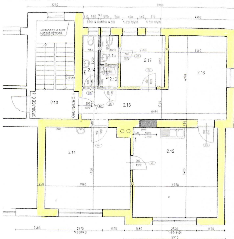
PŮDORYS 2.NP - NOVÝ STAV
