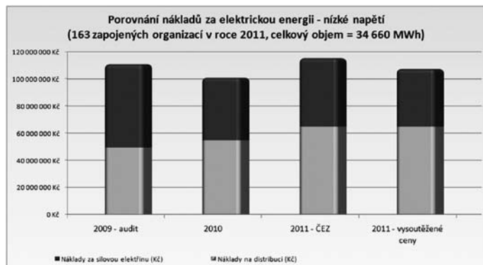
Statutární město Ostrava - Porovnání nákladů za elektrickou energii - nízké napětí
